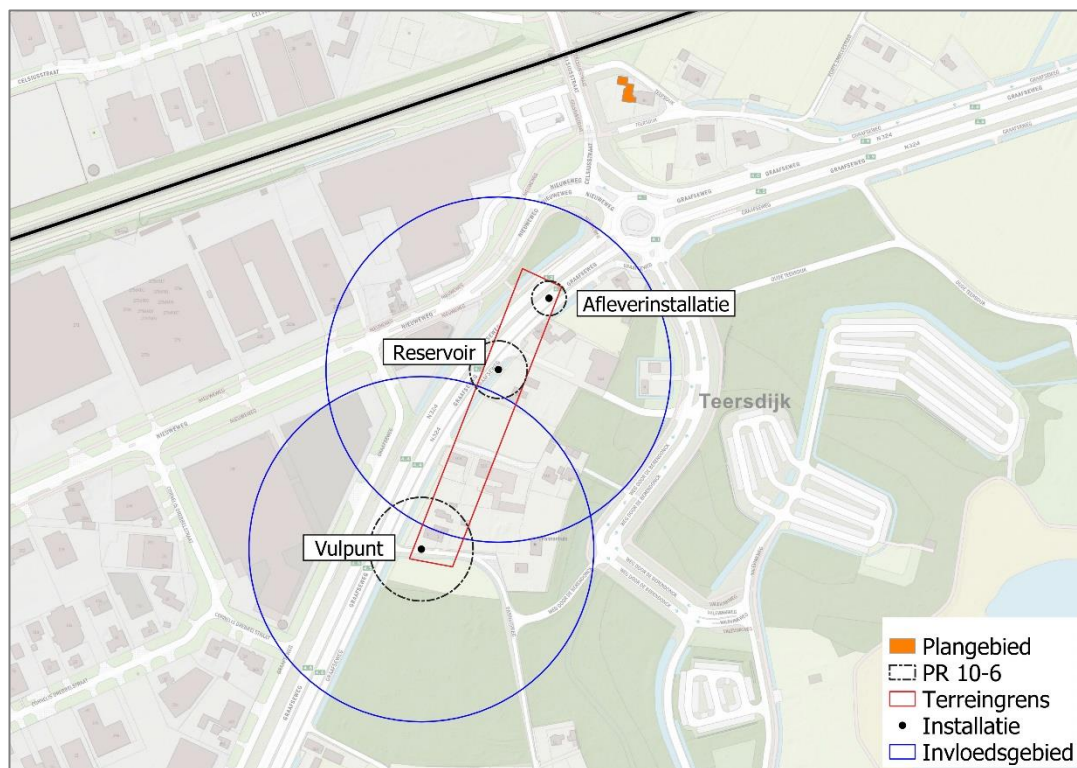
Figuur 3. LPG-tankstation en invloedsgebied
